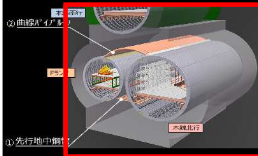
【ステップ⑤】 切詰めセグメント設置工・背面充填工
